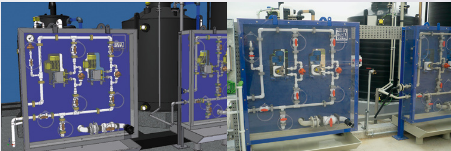
Diseño 3D de Panel para descarga de productos químicos a Tanque de almacenamiento (izquierda) y foto del panel construido (derecha) 3D design of a Panel for discharge of chemical products to the tank (left) and photograph of the panel as built
